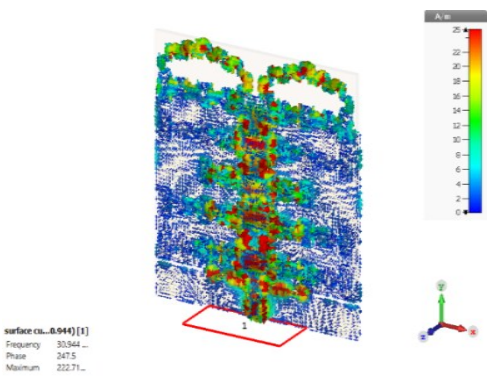
(d) State-4 at 30.9 GHz.
